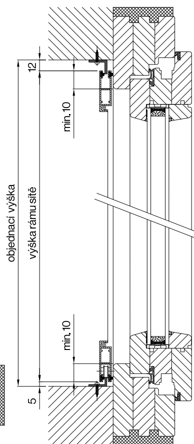
PS LL - svislý řez
