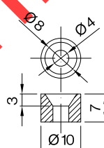
doraz
