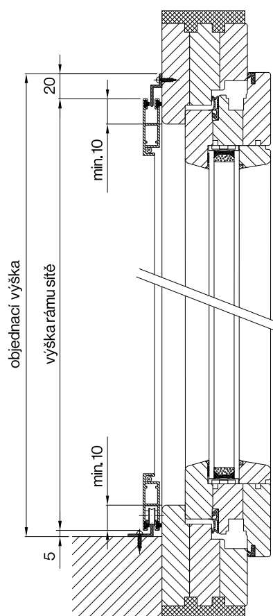
PS ZL - svislý řez
