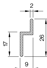
profil Z (horní)
