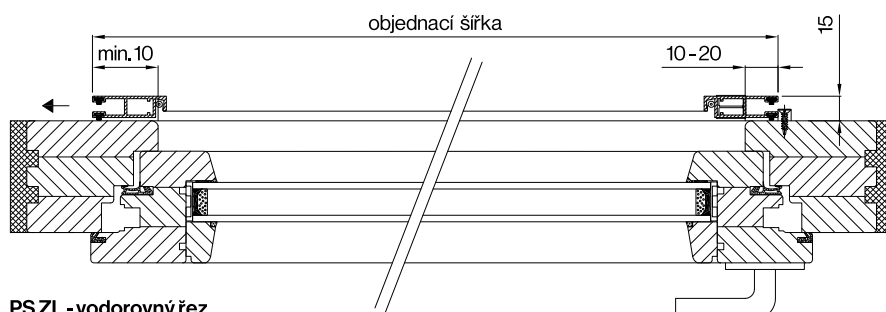
PS ZL - vodorovný řez
