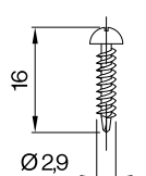
šroub č. 1
