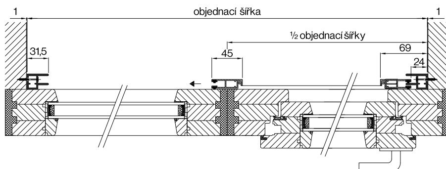
PSR1 - vodorovný řez
