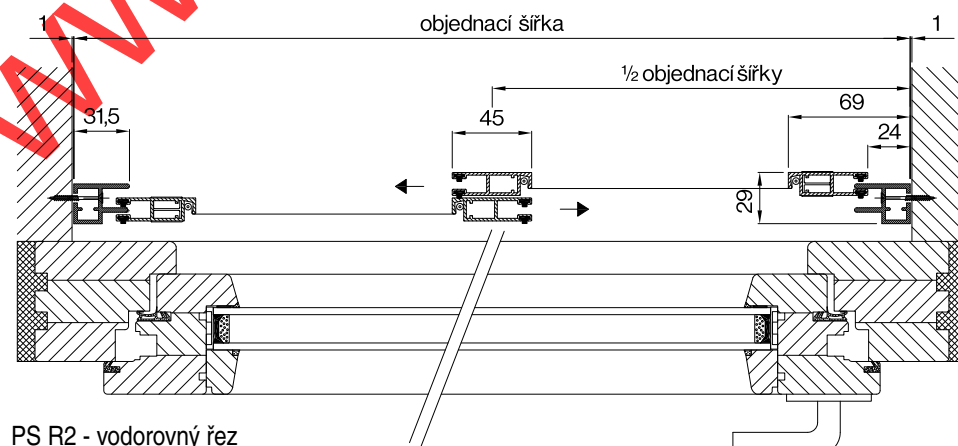
profil R
