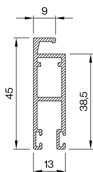
profil rámu sítě
