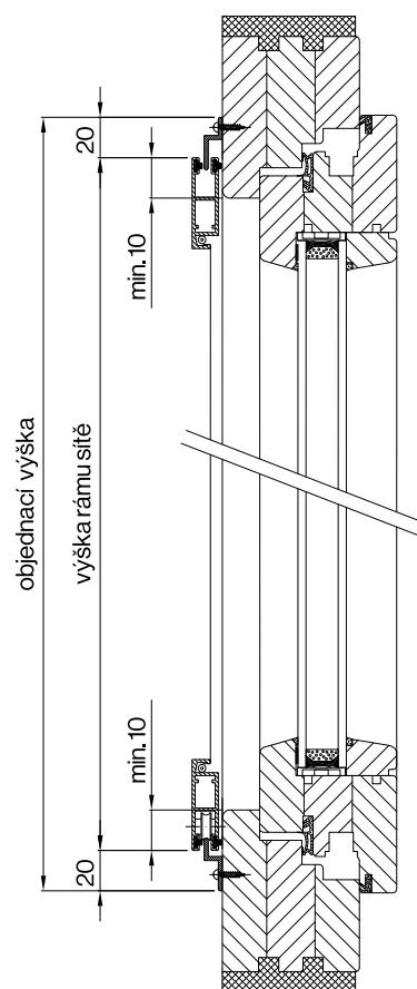
PS Z - svislý řez
