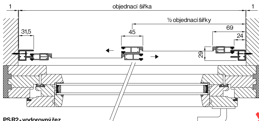
PSR2 - vodorovný řez
