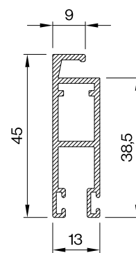
profil rámu sítě
