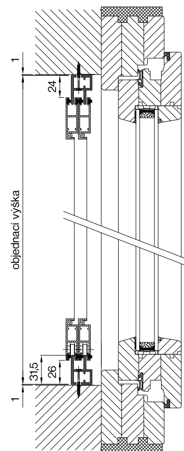
PS R2 - svislý řez
