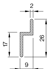
profil Z (horní)
