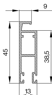
profil
