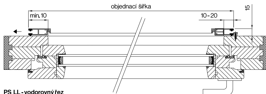
PS LL - vodorovný řez
