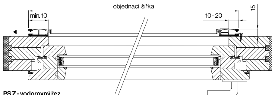
PSZ - vodorovný řez
