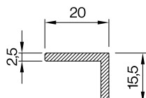
profil L15 (horní)
