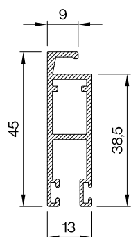
profil rámu sítě
