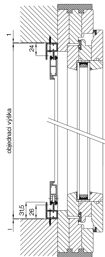
PS R1 - svislý řez
