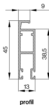
profil
