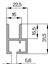
profil R
