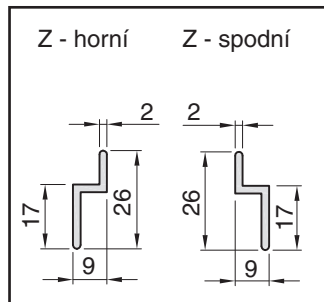
Řezy lišt Z, Z
