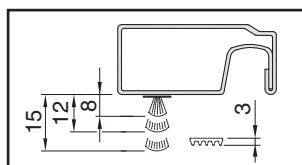
Možnost samolepící těsnící kartáček nebo guma (příbaleno)
