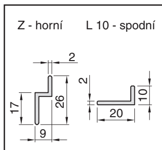
Řezy lišt Z, L
