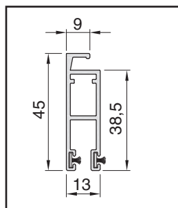
Řez profilem křídla sítě
