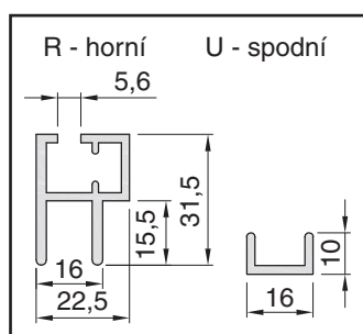
Řezy lišty R, U
