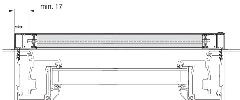
Vodorovný řez - montáž na rám
