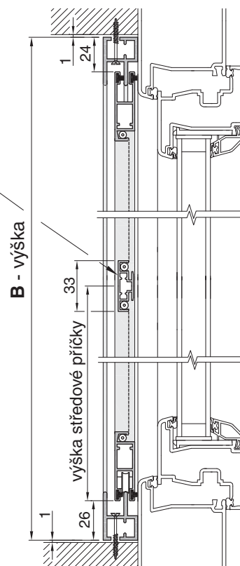
Svislý řez
