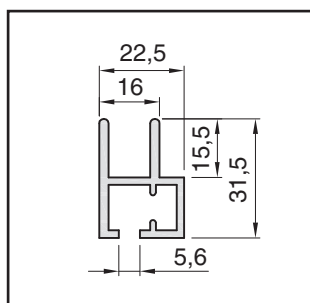
Řez rámu R
