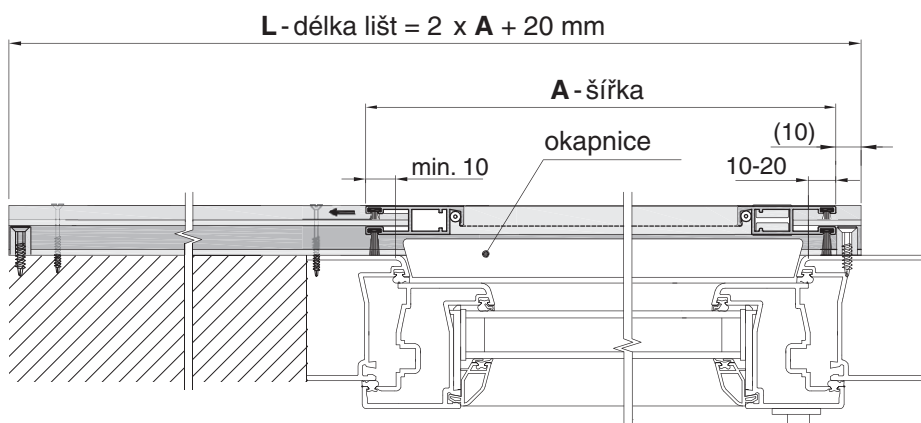
Vodorovný řez
