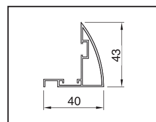
Řez L profilem
