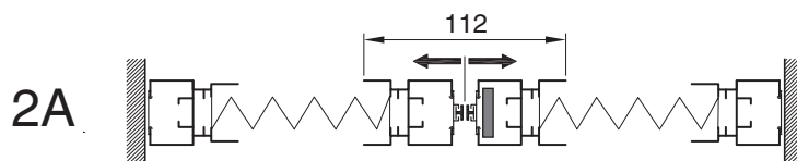
dvoukřídlé - zavírání do středu
