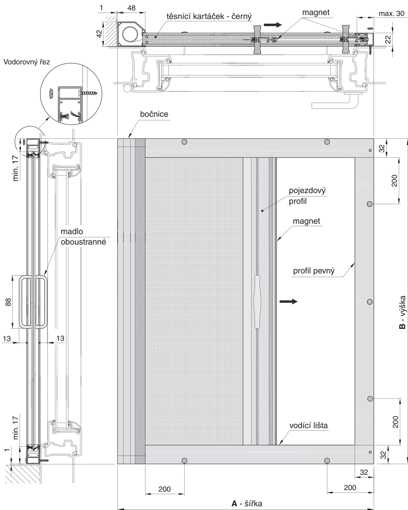
Svislý řez
