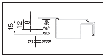
Možnost samolepící těsnící kartáček nebo guma (přibaleno)
