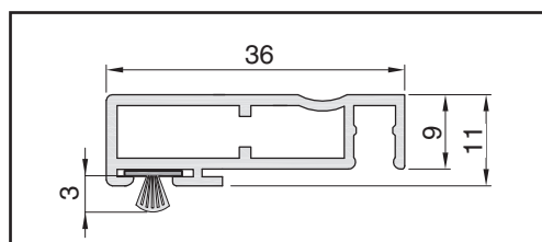
Řez profilem 36 mm
