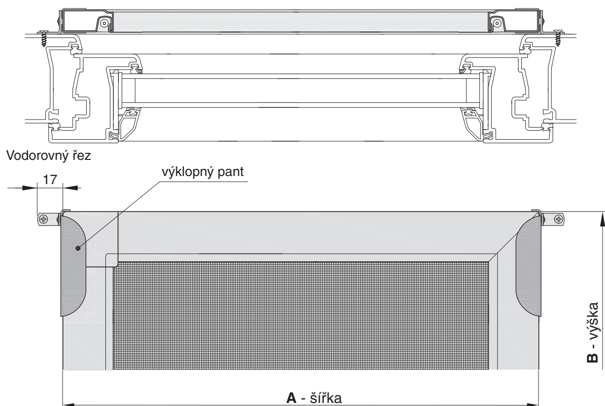
Pohled z exteriéru
