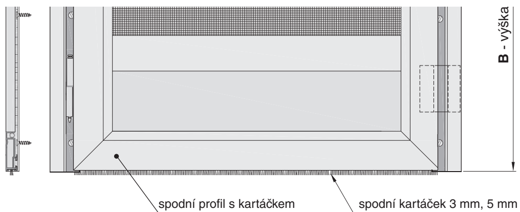
Pohled z montážní strany - provedení bez spodní části rámu - spodní kartáček
