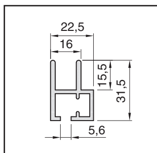
Řez lišty R
