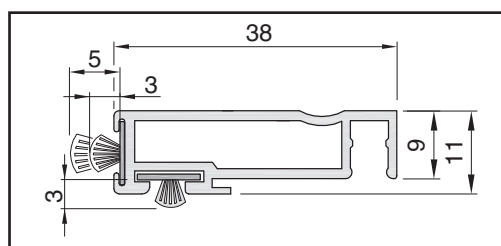
Možnost profilu s těsnícím kartáčkem (provedení s obrtlíky)
