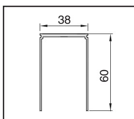
Řez horním profilem
