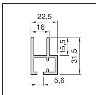
Řez rámu R
