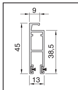
Řez profilem křídla sítě
