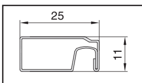
Řez profilem 25 mm
