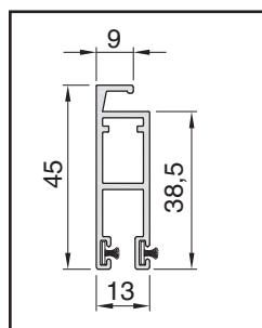
Řez profilem křídla sítě
