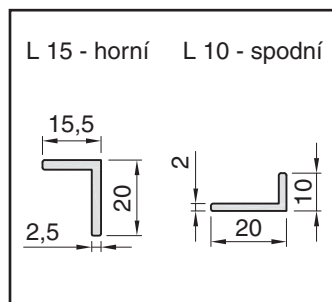
Řezy lišt L, L
