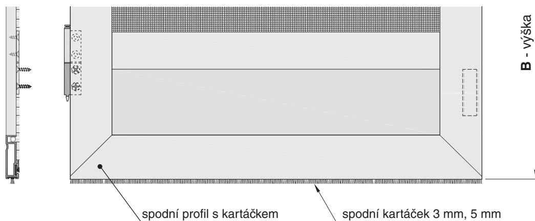
Pohled z montážní strany - provedení spodní kartáček
