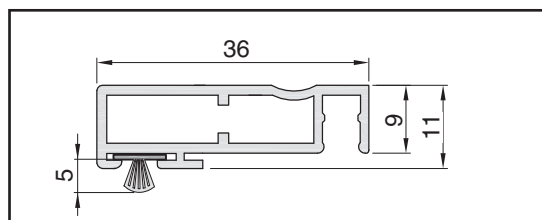
Řez profilem 36 x 11 mm EXTRA
