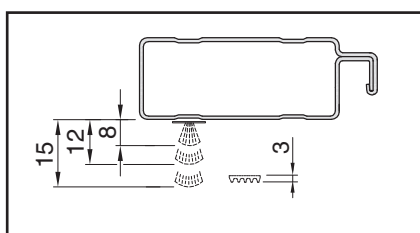
Možnost samolepící těsnící kartáček nebo guma (přibaleno)
