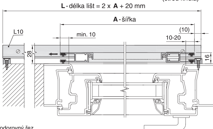
Vodorovný řez
