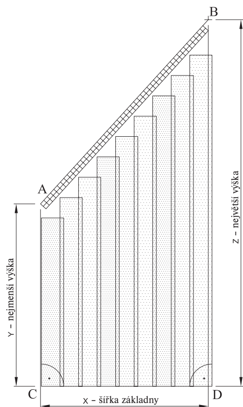
Vertikální žaluzie Blue Line – rozměry šikmého provedení, Obrázek č. 24
