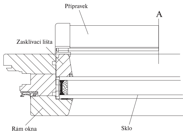
Přiložení přípravku a označení rysky A, Obrázek č. 16
