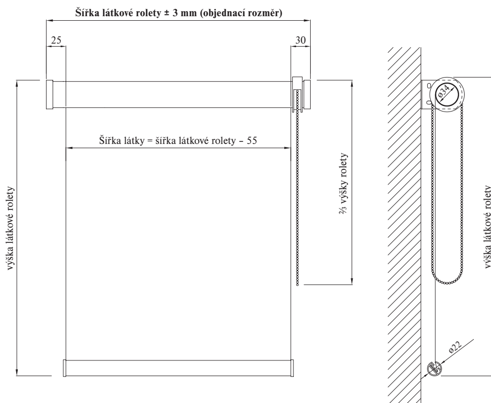
Vnitřní látková roleta Apollo – ovládání řetizek, Obrázek č. 11
