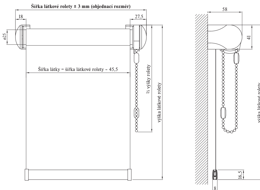
Vnitřní látková roleta Calypso – ovládání řetizek, Obrázek č. 12
