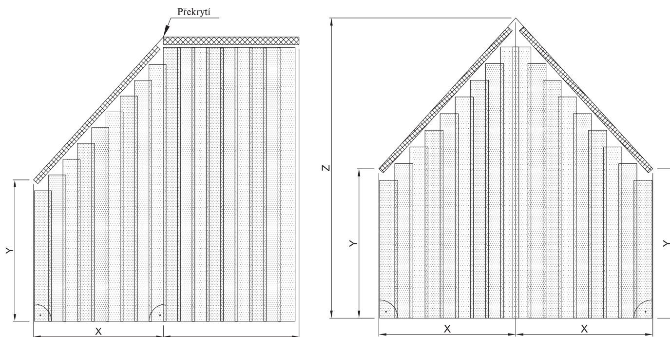
Vertikální žaluzie Blue Line – příklady šikmého provedení, Obrázek č. 25
