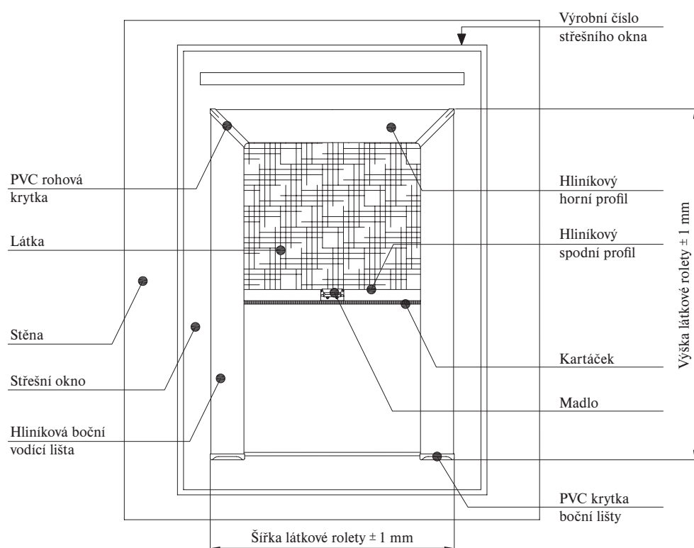
Vnitřní látková roleta Titan – čelní pohled, Obrázek č. 14
