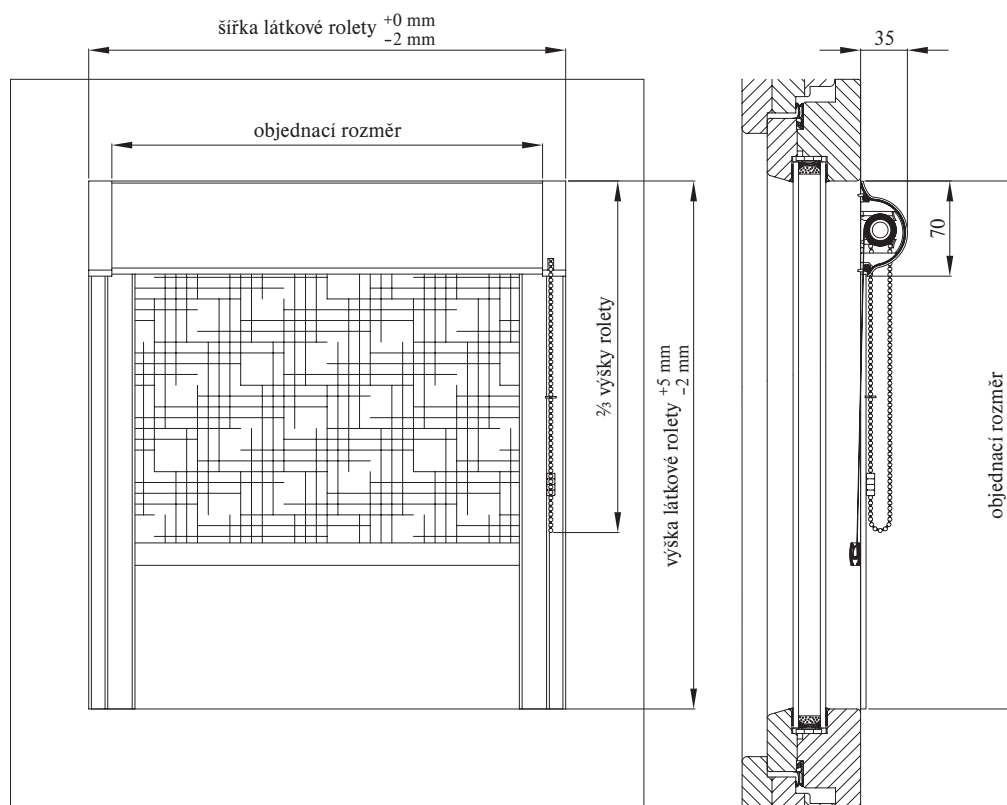
Vnitřní látková roleta Orion – ovládání řetězek, Obrázek č. 13
