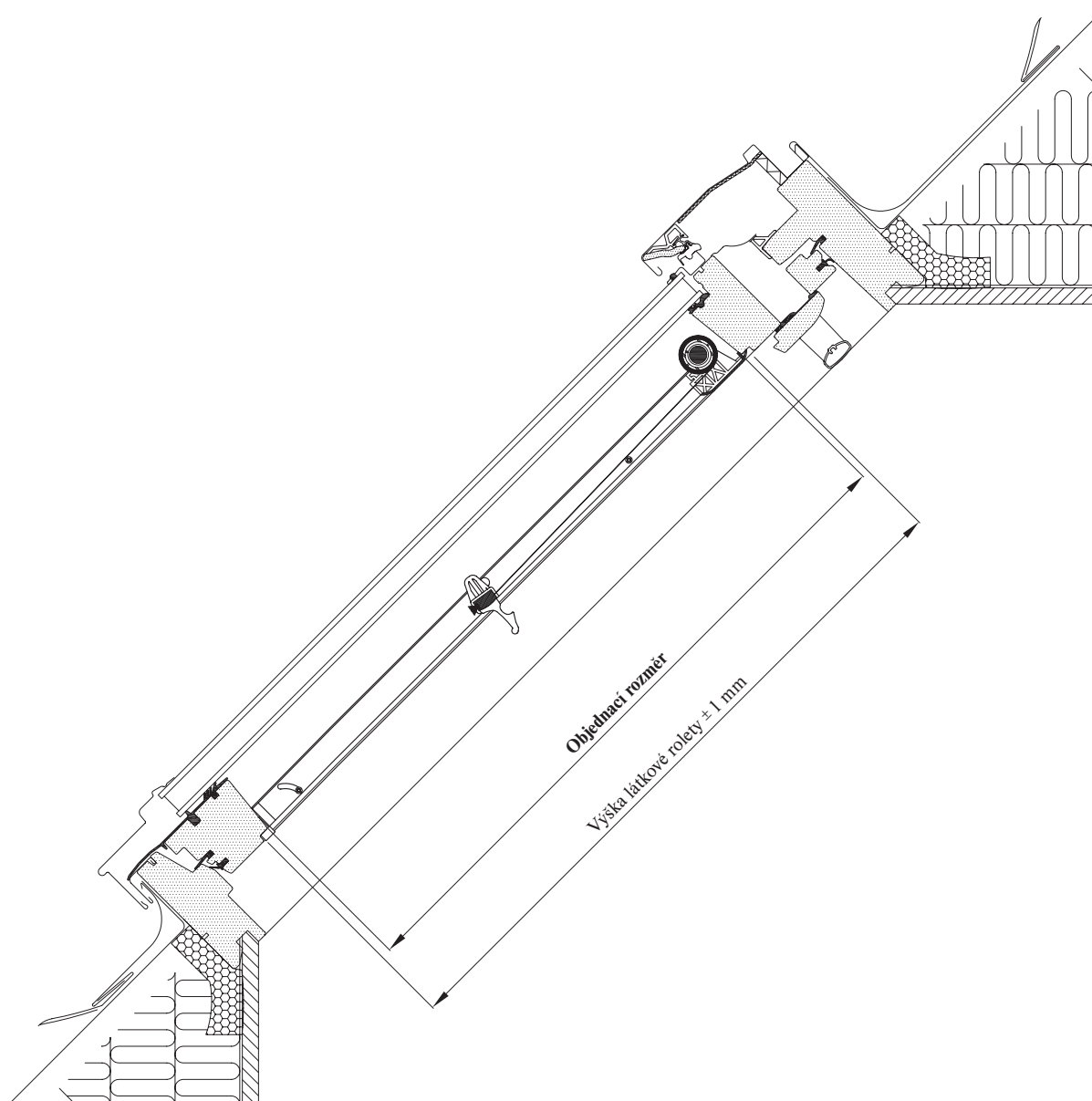
Vnitřní látková roleta Titan – podélný a svislý řez, Obrázek č. 15
